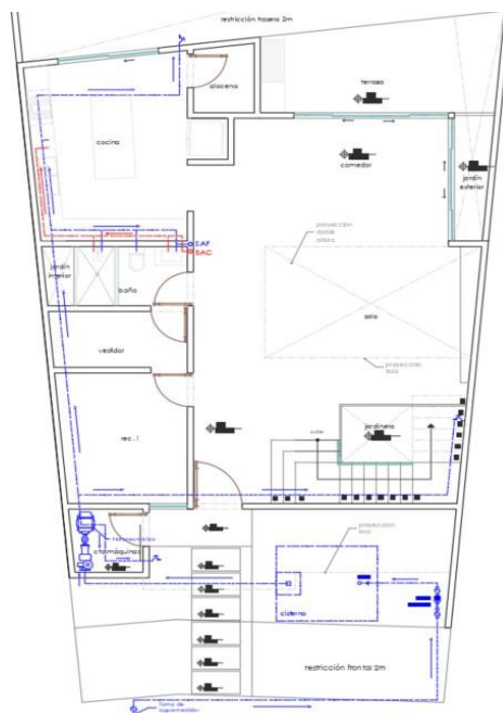
PLANTA BAJA Instalación Hidráulica
