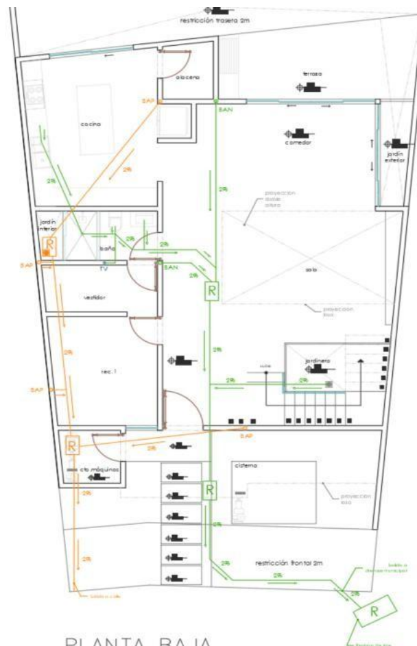
PLANTA BAJA Instalación Sanitaria-Pluvial
